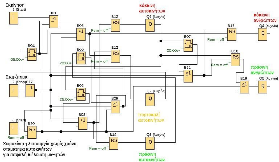
Διάγραμμα Κυκλώματος φαναιρών δρόμου Πρόγραμμα σε FBD Logo
